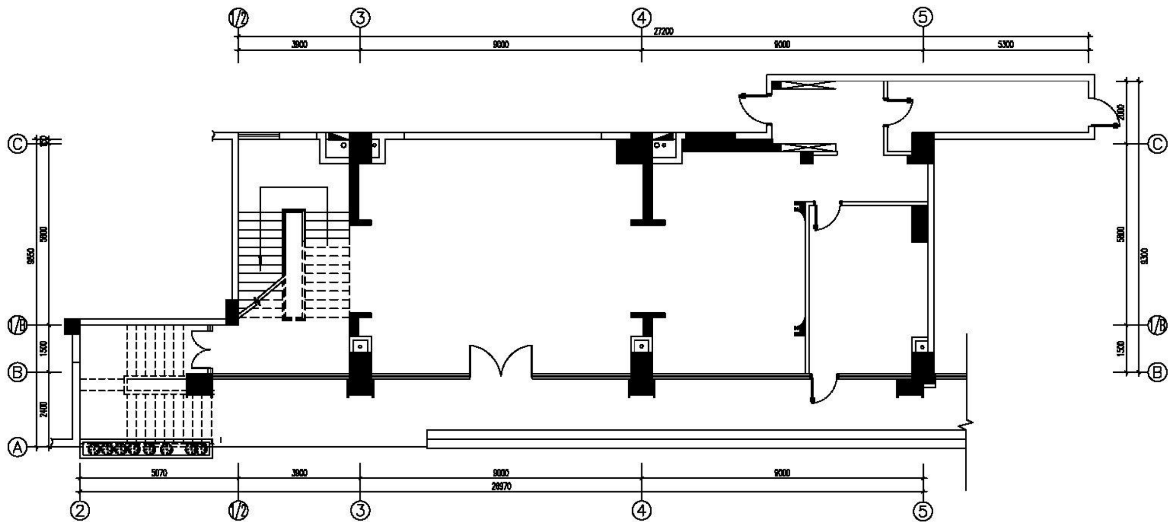
B座西侧一楼平面图
